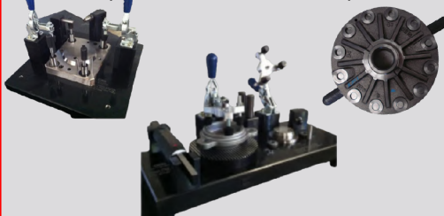
CALIBRES PARA CONTROL DE POSICION VERDADERA (TRUE POSITION GAGE)
